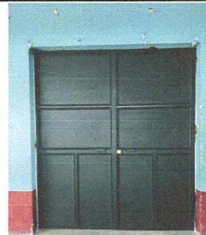
Foto 6: Mejoramiento de 7 puertas que ya se encuentran deterioradas y asi mismo brindar una mejor seguridad a los modulos del establecimiento.
